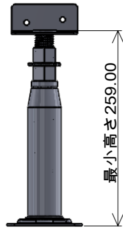
正面最小 スケール1/5
