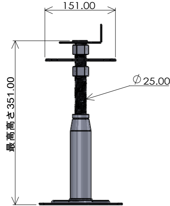
側面最大 スケール1/5
