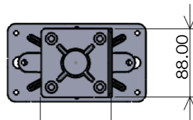
側面最大 スケール1/5
