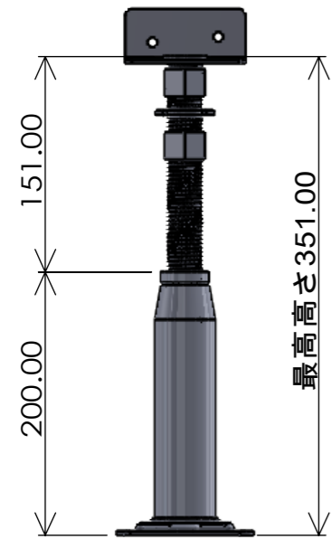
正面最大 スケール1/5
