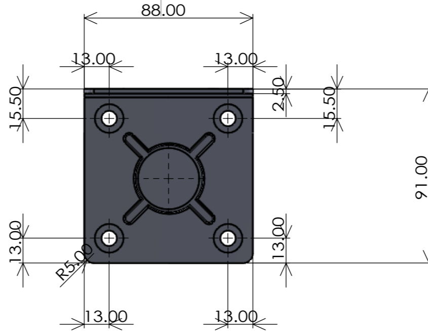
穴寸法 スケール1/2
